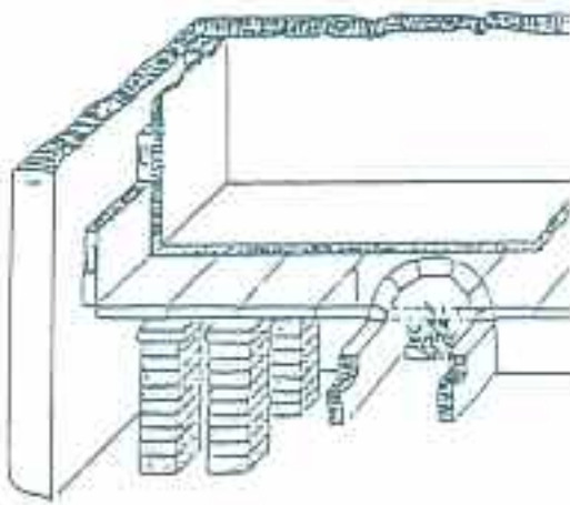
Εικόνα 5: Σχεδιαστική απόδοση υποκαύστων. (Αρχείο ΥΠΠΟ)
